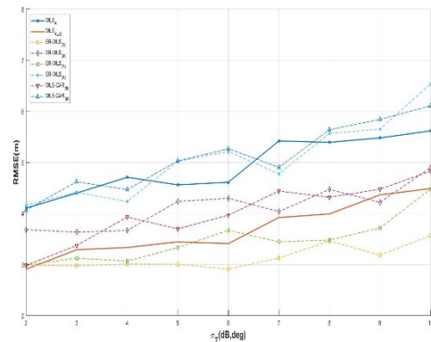
شکل ۶: RMSE برحسب \delta_T (dBm, deg) جایبکه N_A = 3 ، N_B = 4 و \delta_{i1} = 0,10 (dBm)
