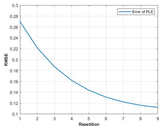
شکل ۴: نمایش RMSE PLE برحسب تعداد تکرار جاییکه N_A = 4 و \delta_{n_{ij}} = \delta_{m_{ij}} = \delta_{v_{ij}} = 10 \text{ (dBm, deg)} ، N_B = 3 ، \delta_{l_i} = 10 \text{ (dBm)}
