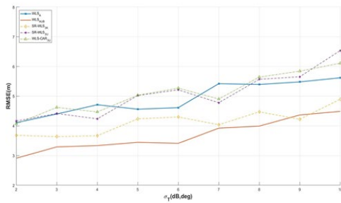
شکل ۷: RMSE برحسب \delta_T (dBm, deg) جایبکه N_A = 3 ، N_B = 4 و \delta_{i1} = 0,10 (dBm) در مقایسه با سایر روشهایی که فقط سه سنسور با مکان معلوم دارند.
