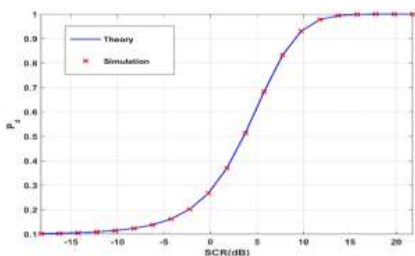
شکل (۲): مقایسه احتمال آشکارسازی تئوری با شبیه‌سازی با فرض P_{fa} = 0.1 و \theta = 45^\circ RCS شناخته شده و \theta = 45^\circ و P_{fa} = 0.1
