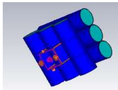
شکل (۱۷): تحقق ساختار بازتابنده پلاسمایی تیغه‌ای با استفاده از لوله‌های افقی و عمودی.
