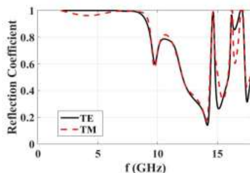
شکل (۱۸): مقدار ضرایب انعکاس ساختار شکل (۱۷) برای دو قطبش عمودی و موازی.
