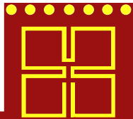
شکل (۳): پیکره‌بندی فیلتر باند باریک پیشنهادی
