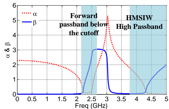
شکل (۶): دیاگرام‌های ثابت انتشار و ثابت تضعیف فیلتر باند باریک پیشنهادی
