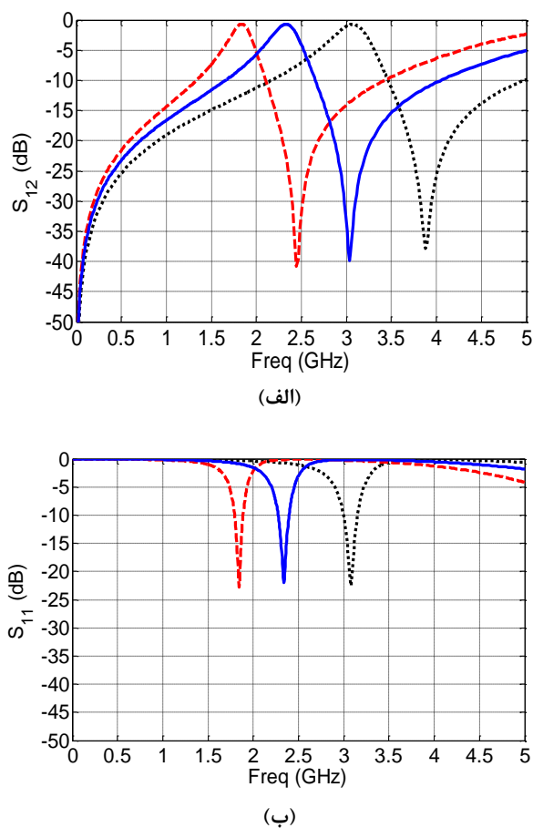
شکل (۵): پاسخ فرکانسی‌های فیلتر باند باریک پیشنهادی با تغییر ابعاد سلول واحد FCSRR. الف) S_{12} و ب) S_{11}
