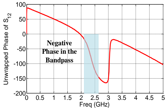
شکل (۸): نمودار فاز فیلتر باند باریک پیشنهادی
