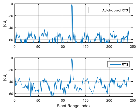
شکل (۱۹): نیم‌رخ برد تصویر دوبعدی پس از فشرده‌سازی در سمت با
