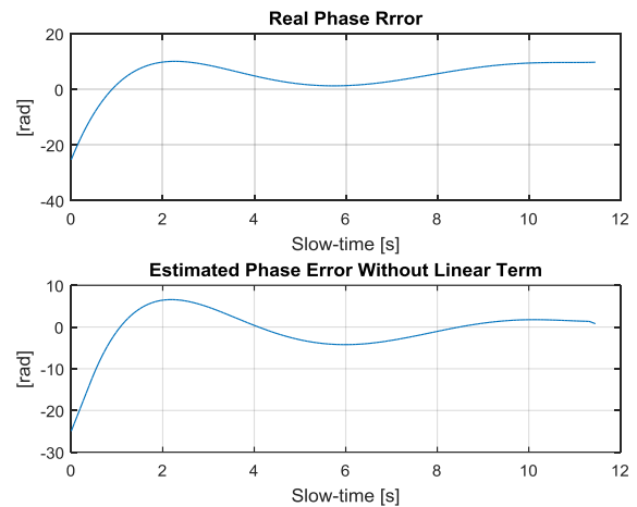
شکل (۱۵): خطای فاز واقعی موجود در سیگنال (بالا) و خطای فاز تخمینی به‌وسیله الگوریتم پیشنهادی (پایین)
