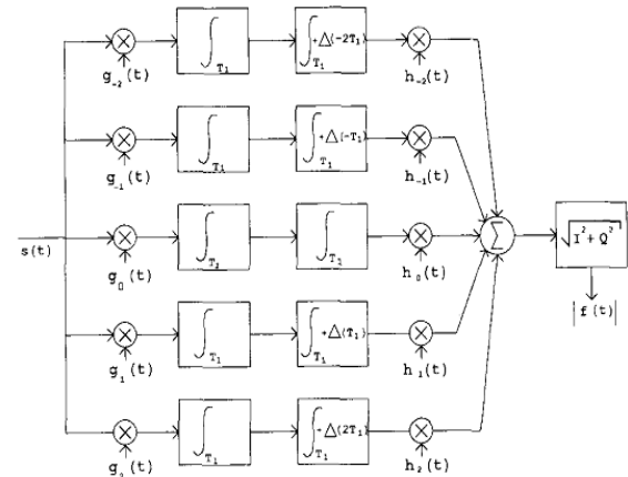
شکل (۲): الگوریتم زیردهانه بی‌درنگ (RTS) [۷]
