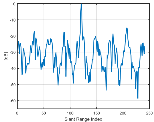
شکل (۱۶): تصویر هدف نقطه‌ای با فرض SNR=0dB پس از
