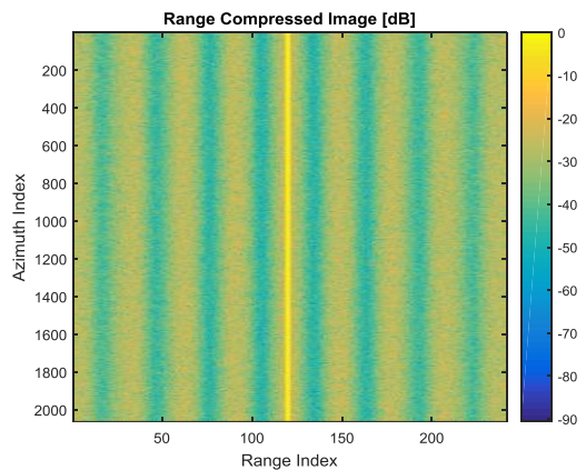
شکل (۱۷): تصویر هدف نقطه‌ای پس از فشرده‌سازی در برد و تصحیح
