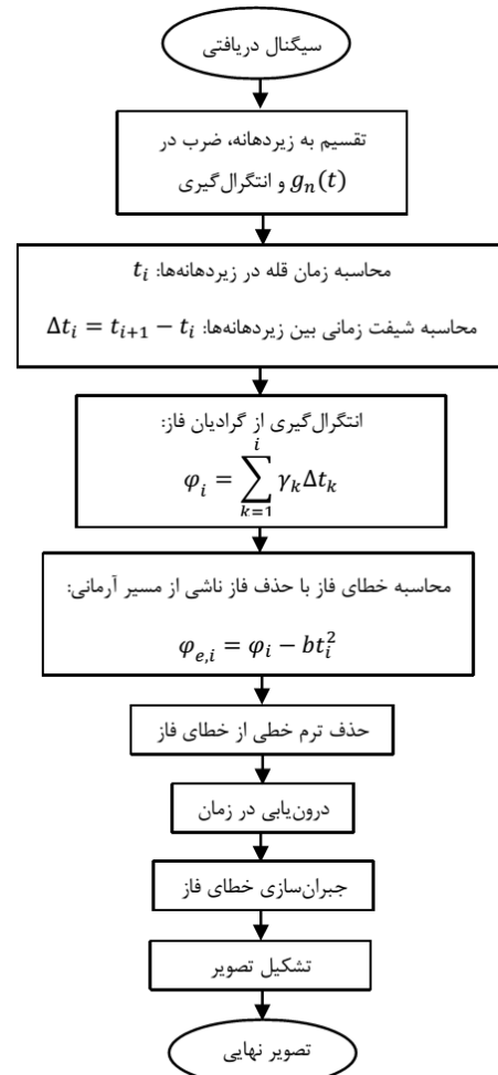
شکل (۴): الگوریتم پایه پیشنهادی برای تخمین خطای فاز
