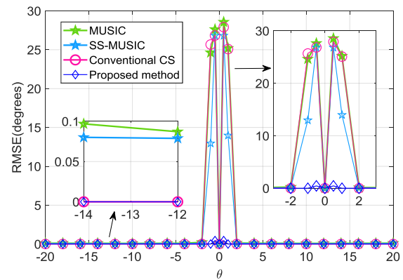
شکل (۶): RMSE بر حسب زاویه به‌ازای یک آرایه خطی غیر یکنواخت با N = 12 آنتن واقعی، 2\ell_N + 1 = 91 آنتن مجازی، K = 2 منبع ارسال‌کننده سیگنال و SNR = -5dB .
