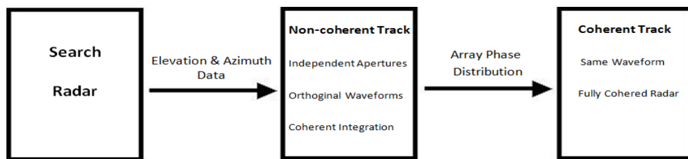
شکل (۱). نمایش بلوکی سیستم SLB کلاسیک
