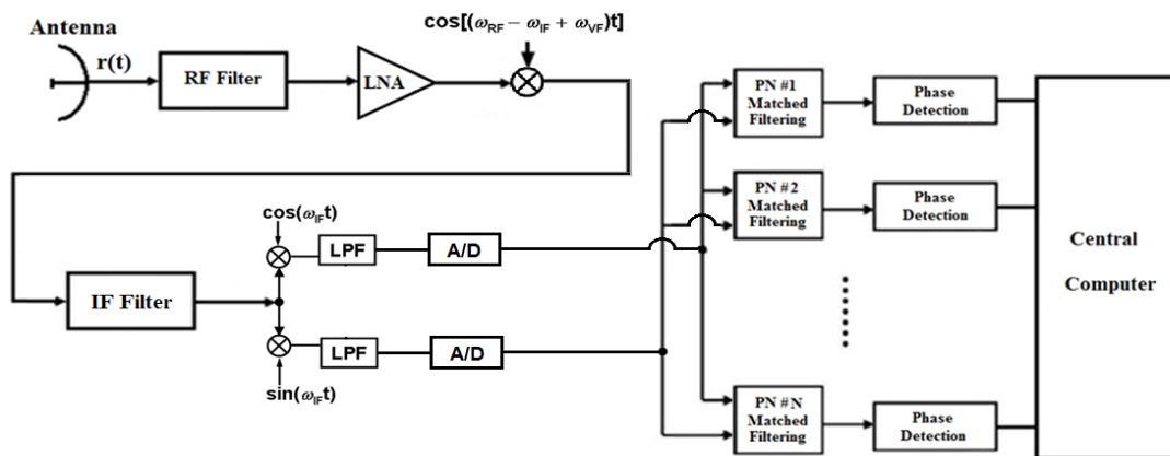
شکل (۳). ساختار ساده‌شده گیرنده.
