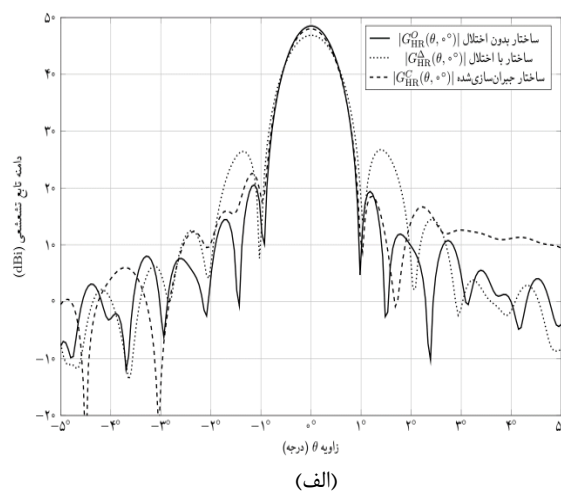
شکل (۱۰). الگوی تشعشی برای آنتن دوبازتابنده ای جبران سازی شده (خط بریده) و آنتن مرجع بدون اختلال (خط ممتد) و آنتن با اختلال (خط نقطه ای). در صفحات اصلی (الف) \phi = 0^\circ و (ب) \phi = 90^\circ ملاحظه می شود که با استفاده از بازتابنده فرعی جبران ساز توصیف شده در شکل (۹) می توان الگوی تشعشی ساختار اختلال یافته را به حالت ایده آل نزدیک نمود.
