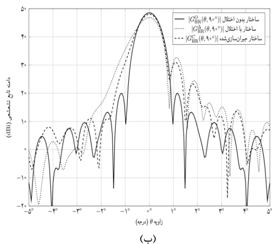
شکل (۱۰). الگوی تشعشی برای آنتن دوبازتابنده ای جبران سازی شده (خط بریده) و آنتن مرجع بدون اختلال (خط ممتد) و آنتن با اختلال (خط نقطه ای). در صفحات اصلی (الف) \phi = 0^\circ و (ب) \phi = 90^\circ ملاحظه می شود که با استفاده از بازتابنده فرعی جبران ساز توصیف شده در شکل (۹) می توان الگوی تشعشی ساختار اختلال یافته را به حالت ایده آل نزدیک نمود.
