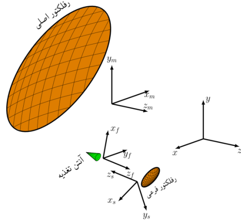
شکل (۱). اجزای مسئله در تحلیل آنتن‌های بازتابنده شامل آنتن تغذیه، بازتابنده فرعی و آنتن تغذیه و دستگاه‌های مختصات مرتبط با هر یک.
