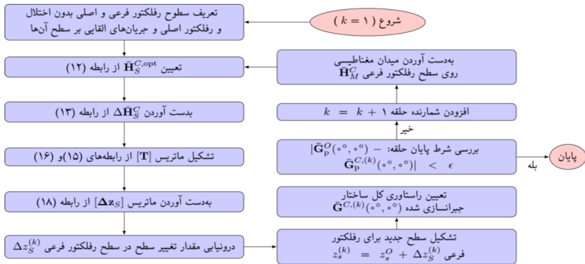
شکل (۴). فلوچارت روش پیشنهادی برای طراحی بازتابنده فرعی جهت جبران سازی اختلال سطح بازتابنده اصلی.
