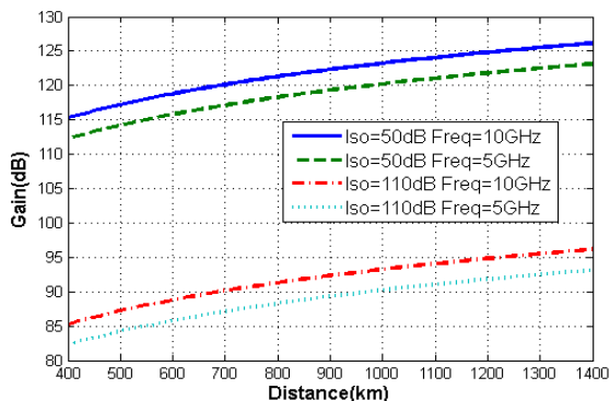
شکل ۳. نتیجه شبهه‌سازی برای رادار فضایی
