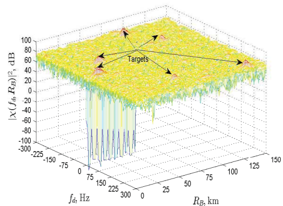
شکل ۱. خروجی تابع ابهام بعد از اعمال روش حذف سیگنال‌های تداخلی در کانال مراقبت
