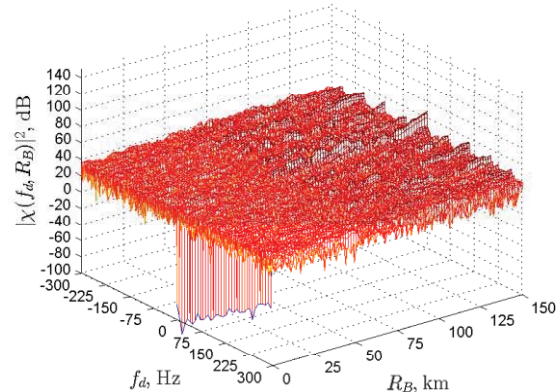
شکل ۷. خروجی تابع ابهام بعد از پاک‌سازی کانال مرجع توسط الگوریتم ST-CMA-RLS و بعد از اعمال روش حذف سیگنال‌های تداخلی در کانال مراقبت در سناریوی ۴ به‌زای کلاتر با طیف توان نامی.
