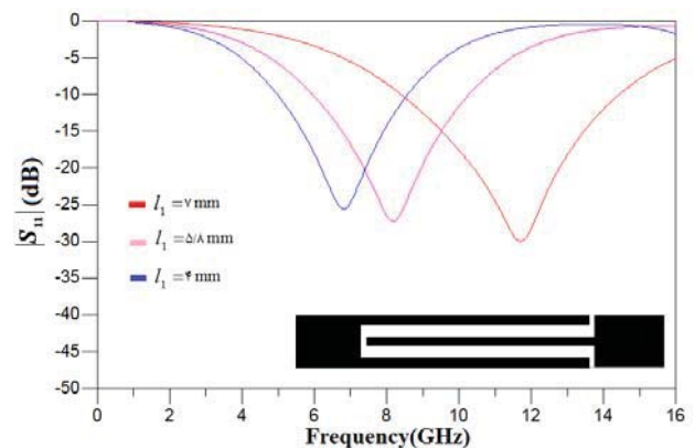
شکل ۶. شبیه سازی پاسخ فرکانسی فیلتر پیشنهادی برای طول خطوط تزویج موازی دوتایی مختلف
