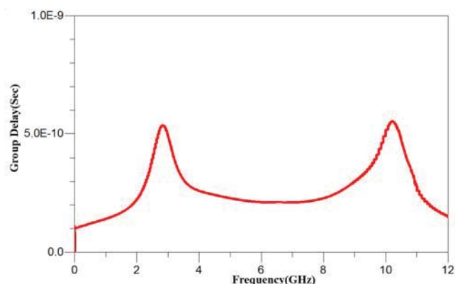
شکل ۱۴. تاخیر گروه شبیه سازی شده فیلتر پیشنهادی
