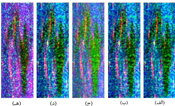
شکل ۸. تصاویر مربوط به روش‌های تجزیه هدف (الف) Freeman-Durdan (ب) Yamaguchi سه جزئی (ج) Yamaguchi چهار جزئی (د) Van Zyl (ه) Krogager
