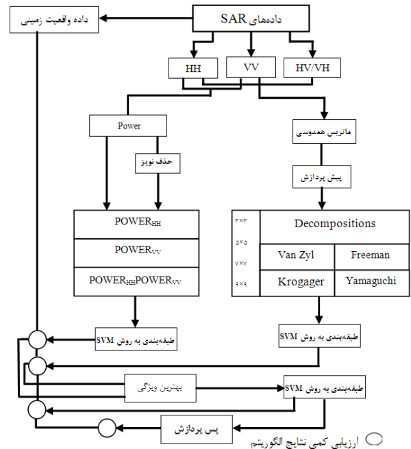
شکل ۲. فلوجارت الگوریتم پیشنهادی جهت آشکارسازی لکه‌های نفتی
