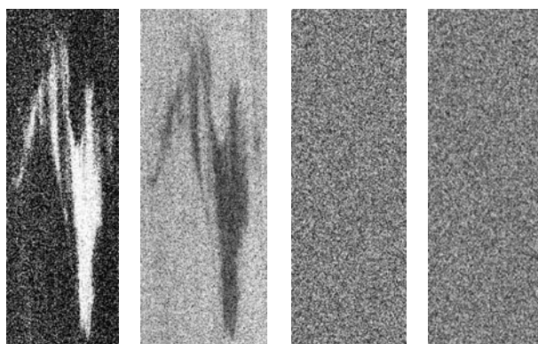
شکل ۳. الف) تصویر مقدار Power پلاریزاسیون HV (ب) تصویر مقدار Power پلاریزاسیون VH (ج) تصویر مقدار Power پلاریزاسیون HH (د) تصویر مقدار Power پلاریزاسیون VV
