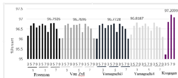
شکل ۹. نتایج طبقه‌بندی ویژگی‌های استخراج‌شده از روش‌های تجزیه
